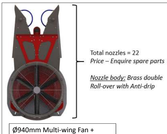
Turret
